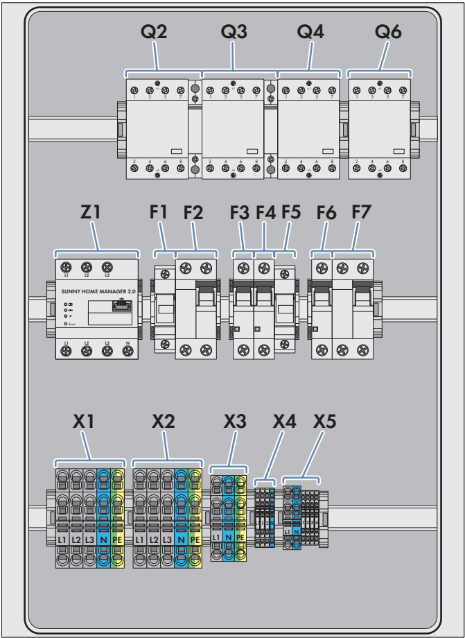
Abbildung 7: Bestückungsvorschlag für 1-phasige Umschalteneinrichtung mit allpoliger Trennung
