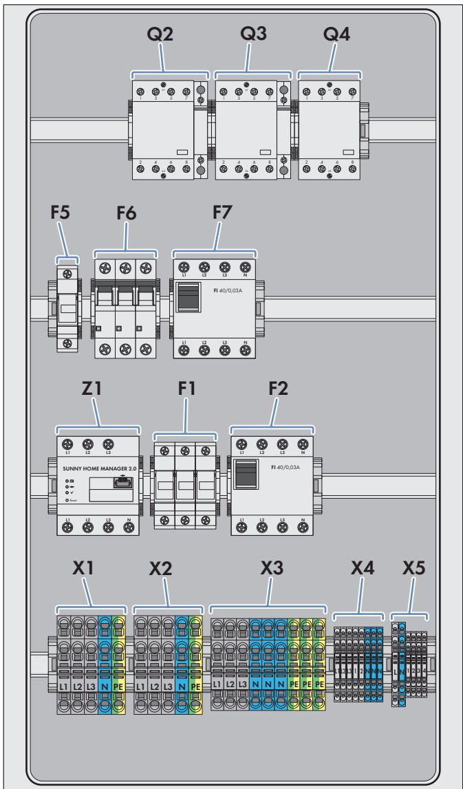
Abbildung 8: Bestückungsvorschlag für 3-phasige Umschalteneinrichtung mit allpoliger Trennung
