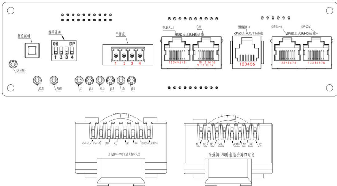
接口板接口示意图
