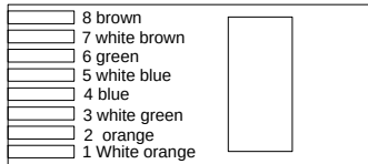
RJ45
