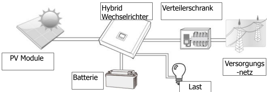
Abbildung 1 Hybrid PV System Überblick
